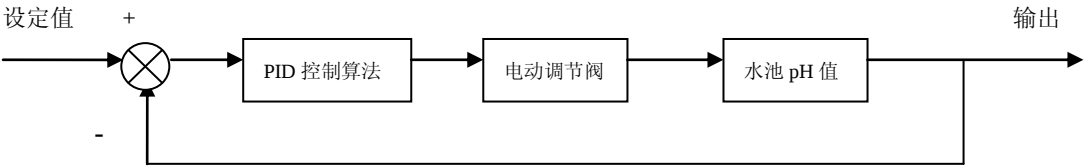
图 3-1 pH 值 PID 控制
