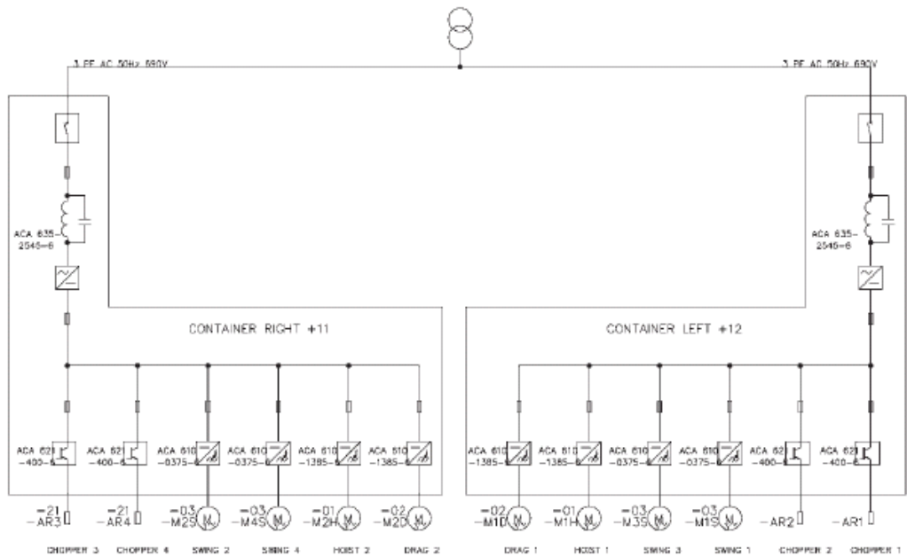
图 2 系统结构图
