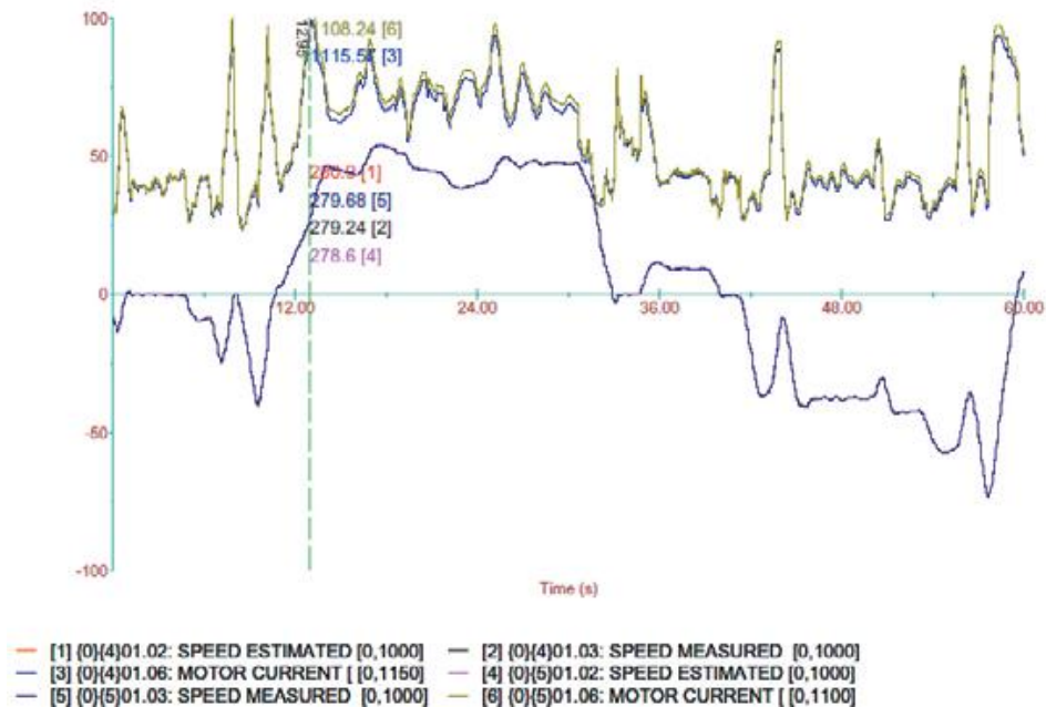
图 3 使用新的交直交驱动技术后的平稳运行
